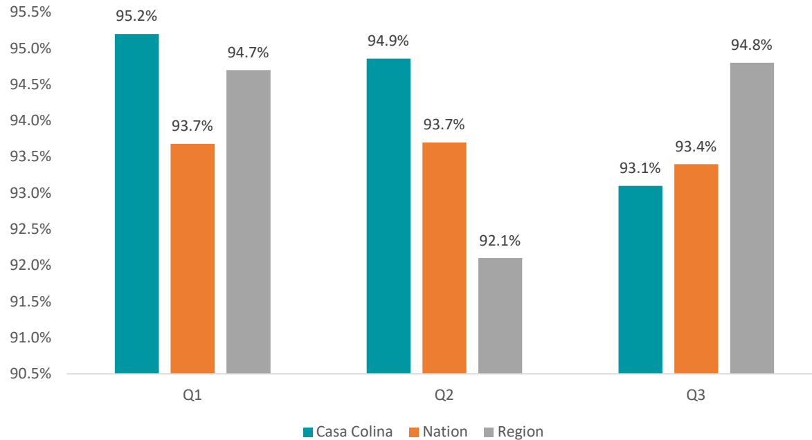
SCI: Individual Therapy Minutes Per Day
