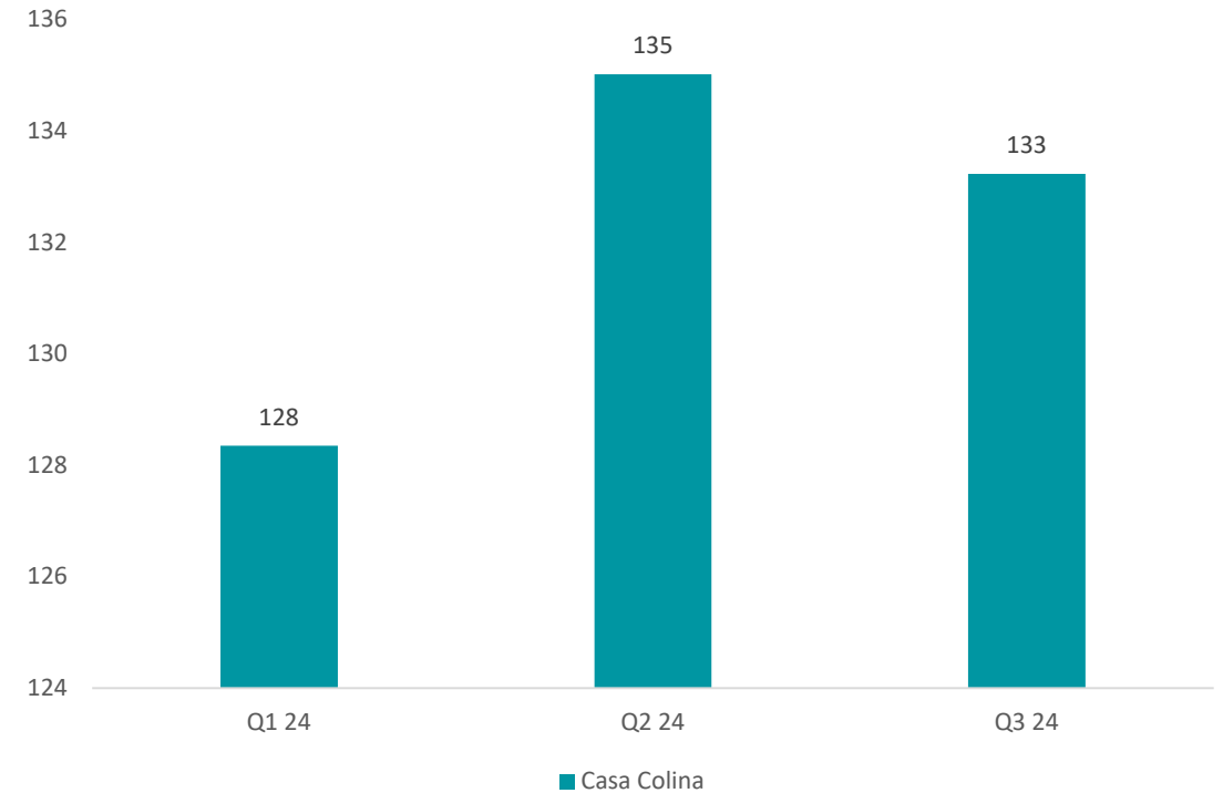
SCI: Total Therapy Minutes Per Day
